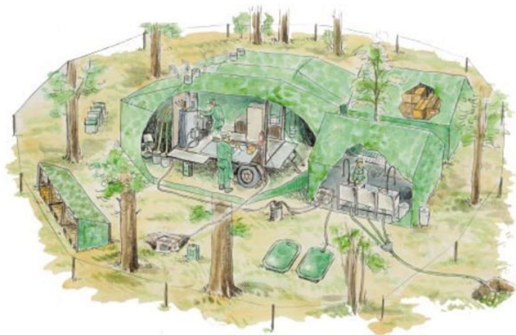
Bild 16. Samgrupperad kokplats med kokutrustning på koktraktorkärra 112 samt diskutrustning och förrådstält
